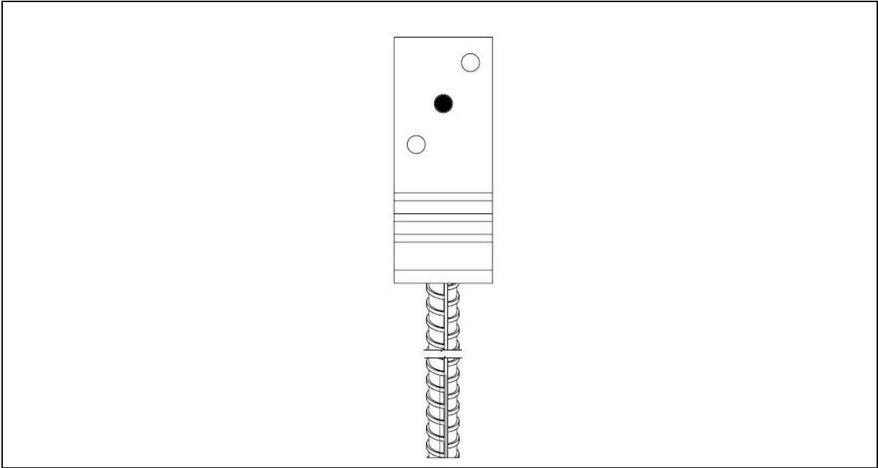
Figure 80 Type PSZ 60, PSZ 70, PSZ 90, PSZ 100, PSZ 120, PSZ 140
