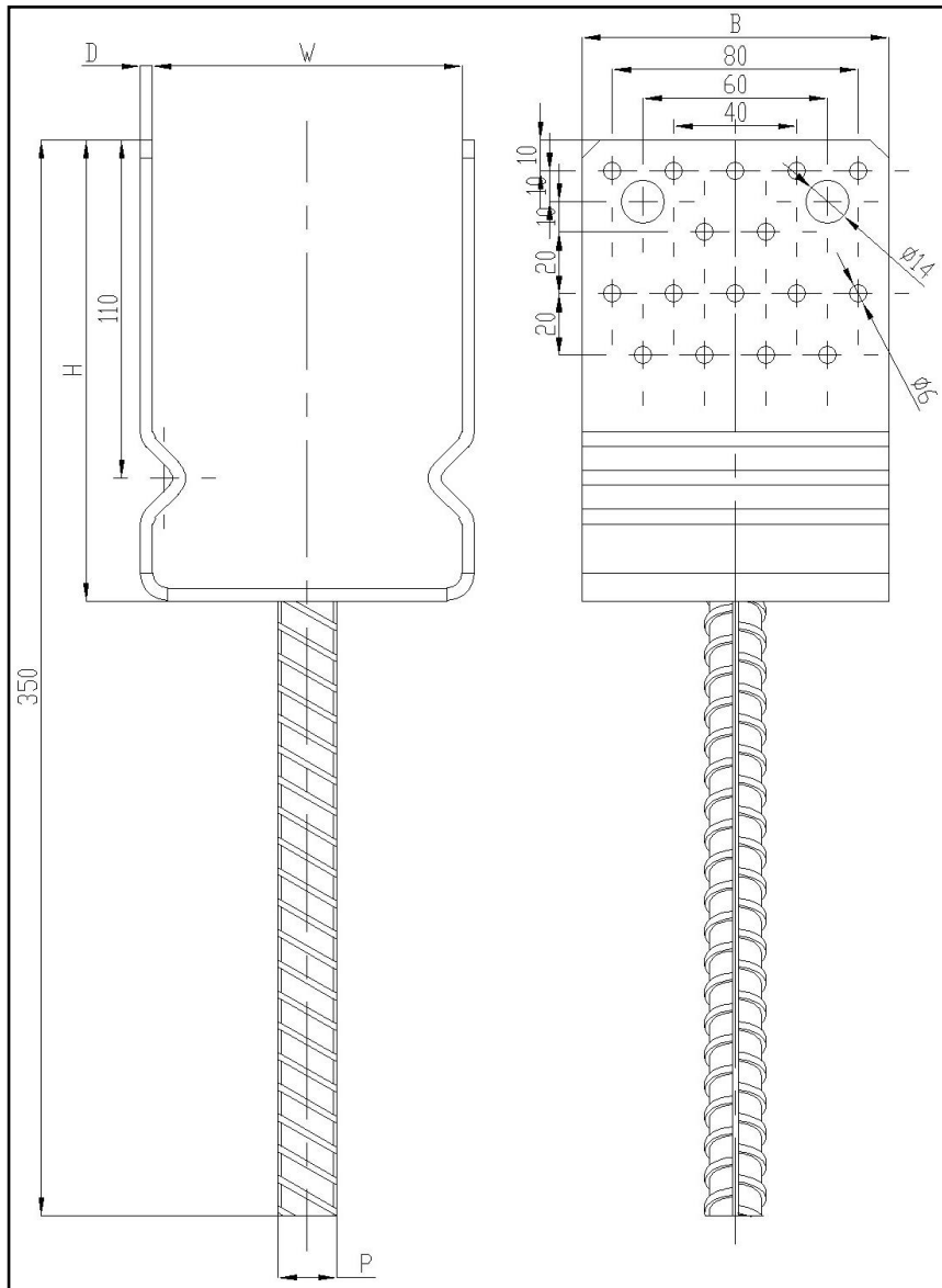
Figure 27 Type PSSZ
